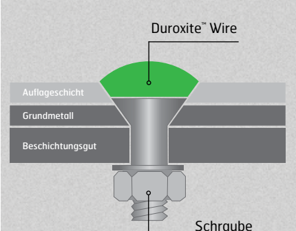
Bolzen von Duroxite™ durch Senkschraubloch
