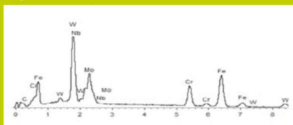
Espectro SEM / EDS que muestra los borocarburos ricos en tungsteno, niobio y molibdeno
