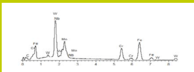
Spectre MEB / SDE présentant des carbures de bore riches en W-Nb-Mo
