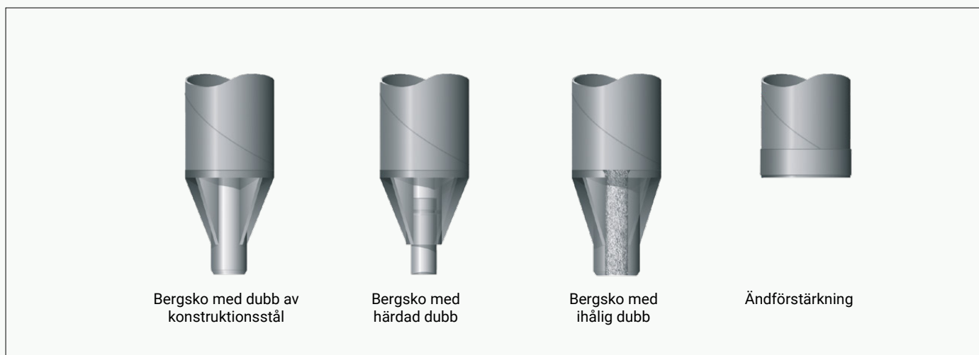
Figur 2.3. Pålskor för grova RR-pålar.
