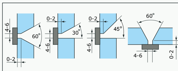
Figur 5.3. Fogtyper för svetsning med rotstöd.
