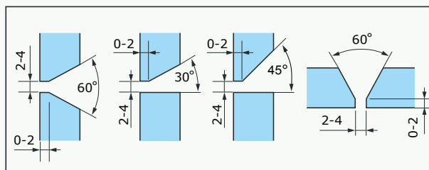
Figur 5.2. Fogtyper för svetsning utan rotstöd.
